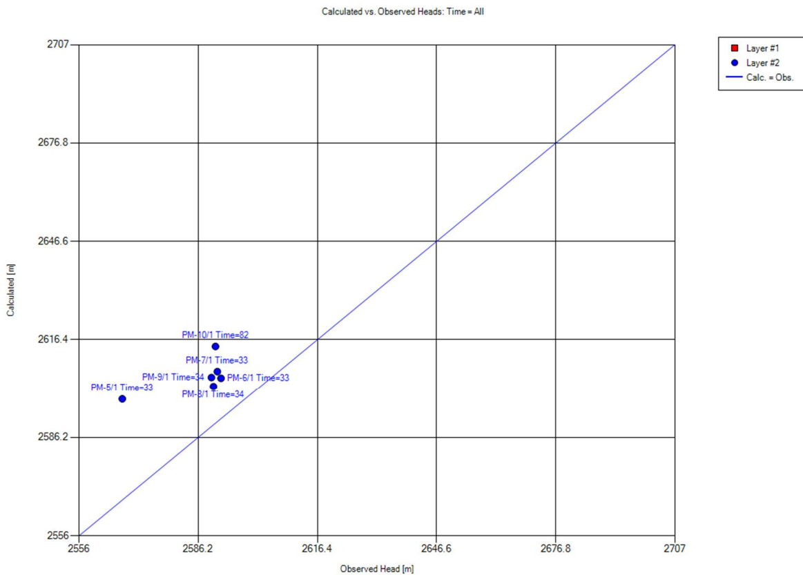
Figura 9: Scatter Plot de los niveles piezométricos calculados vs observados para la validación del modelo utilizando los pozos medidos de junio a julio.
