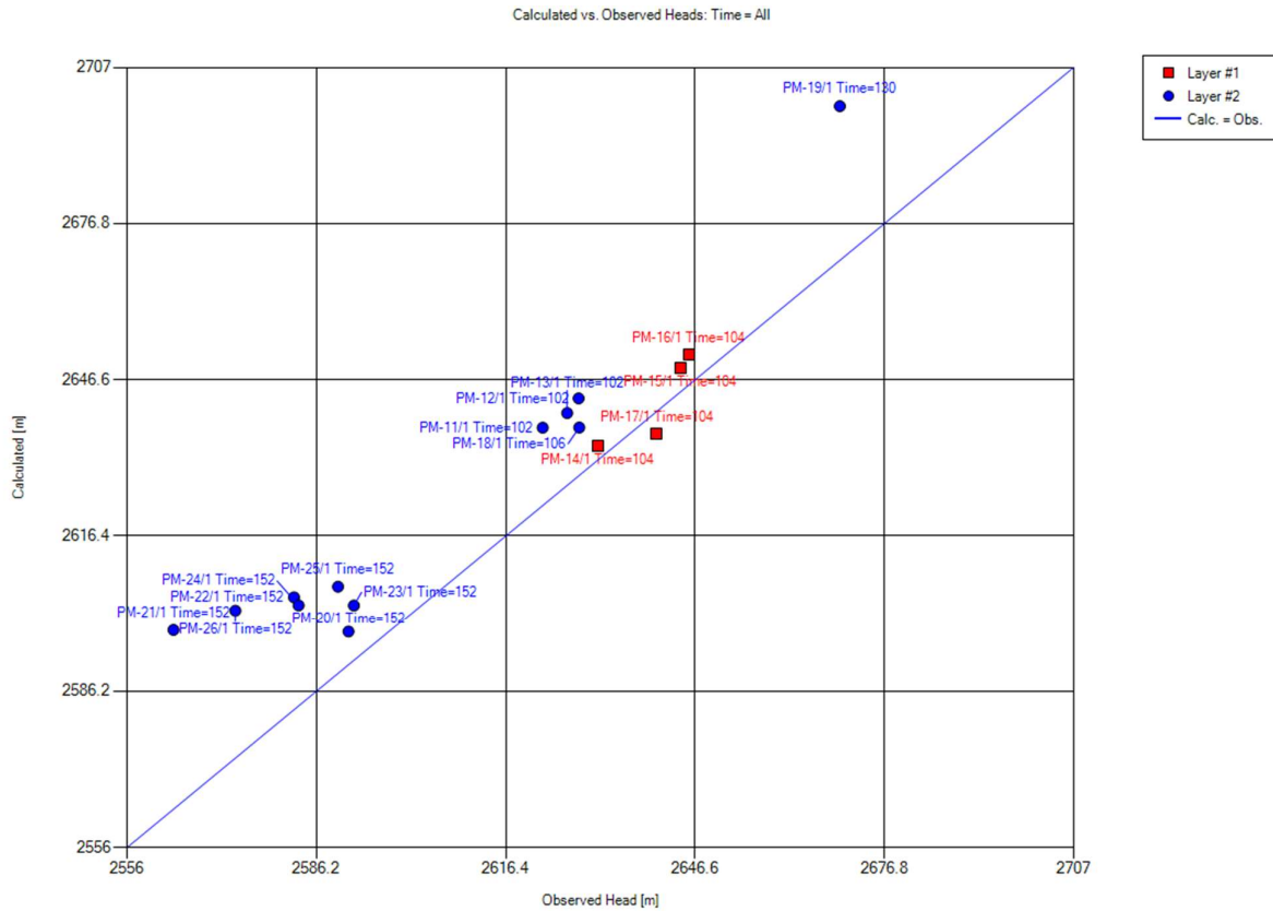
Figura 8: Scatter Plot de los niveles piezométricos calculados vs observados para la calibración final del modelo utilizando los pozos medidos de agosto a septiembre.
