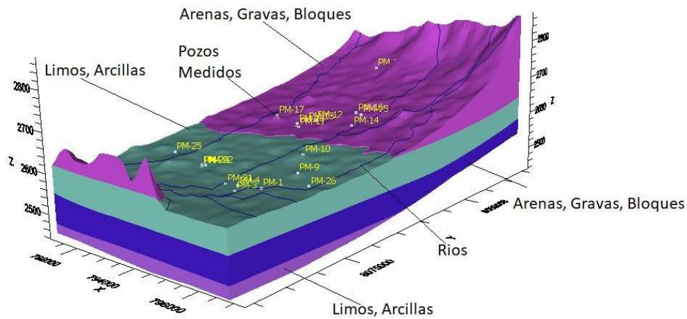
Figura 7: Modelo conceptual de la zona de estudio.
