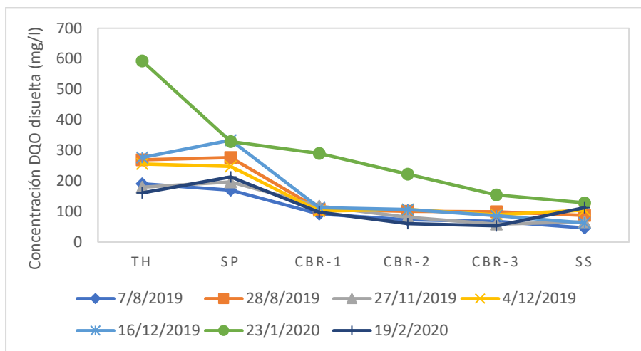
Figura 4 - Variación de la concentración de DQO soluble en el tratamiento.
