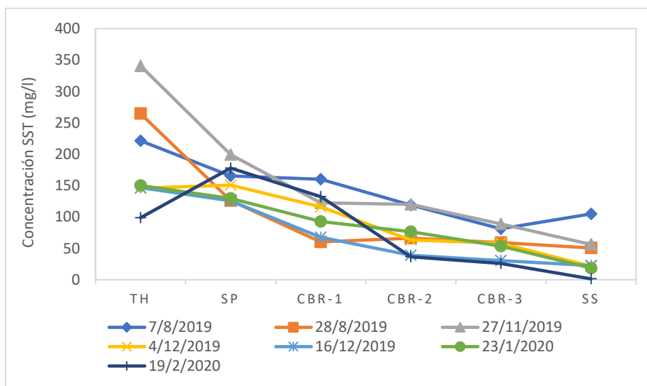
Figura 5: Variación de la concentración de SST en el tratamiento.
