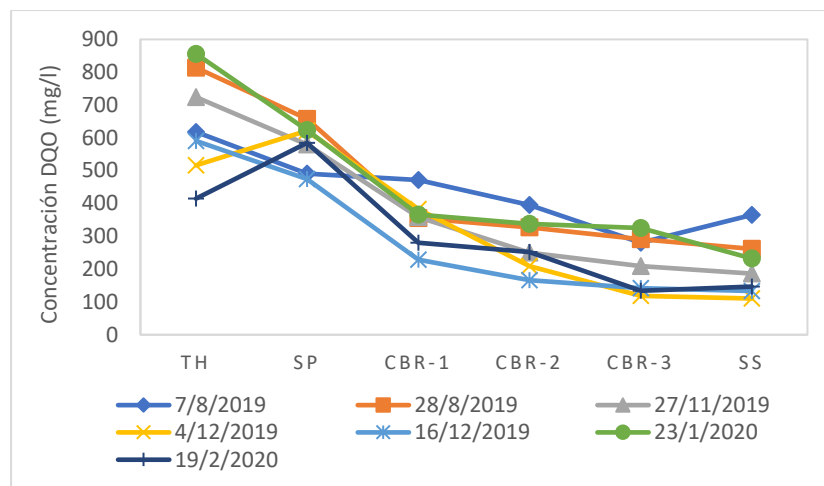
Figura 3 - Variación de la concentración de DQO total en el tratamiento
