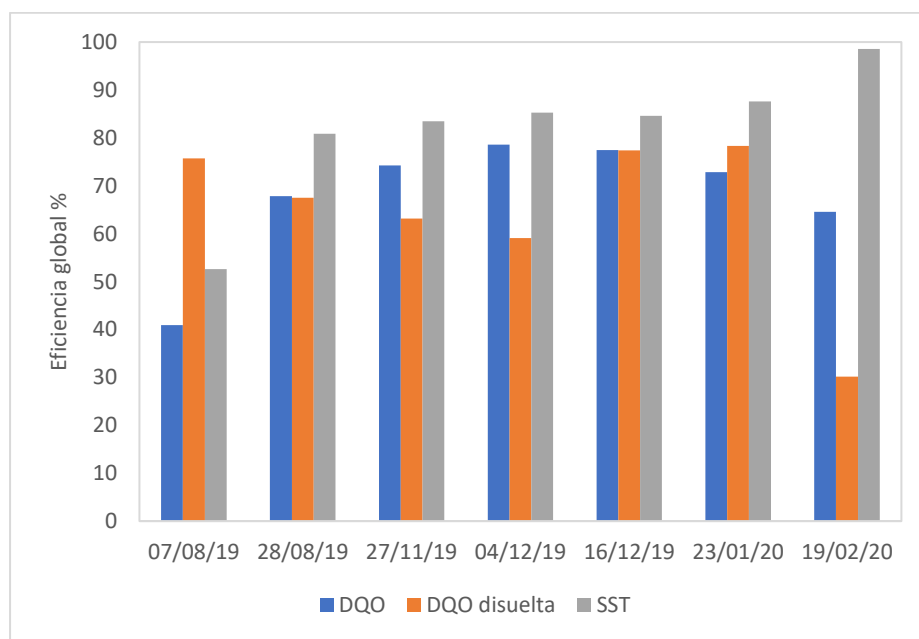
Figura 6: Eficiencia global de la planta piloto.
