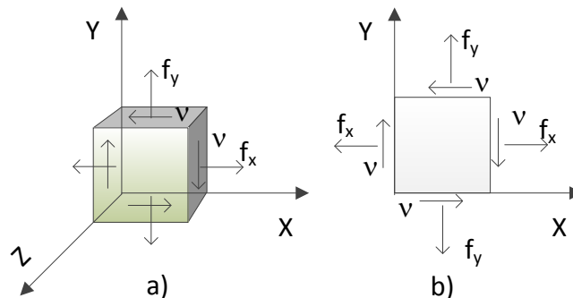
Figura 4 – Tensiones membranales.
