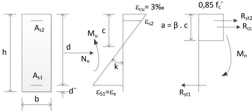
Figura 9 – Diagramas del bloque de tensiones rectangular y deformaciones de la norma ACI.
