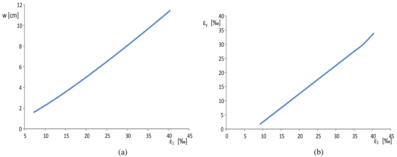
Figura 13 – Curvas mostrando la variación de w con \varepsilon_1 y de \varepsilon_y con \varepsilon_1 .
