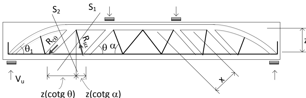
Figura 1 – Modelo de cercha discreta generalizada que es la estructura resistente de una viga sujeta a flexión y cortante.
