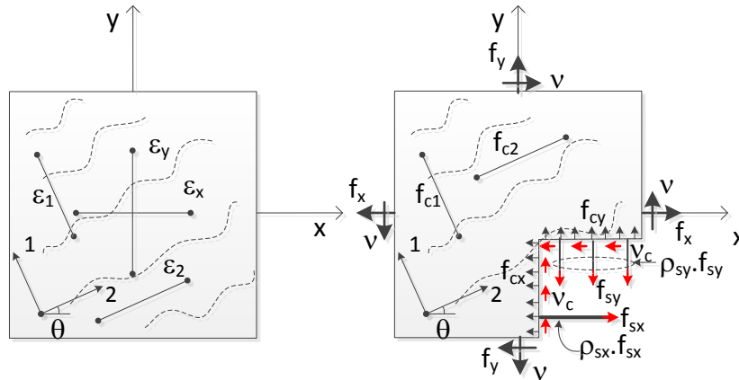
Figura 6 – Elemento de un panel de hormigón sujeto a tensiones y deformaciones medias (adaptada de Aguirre [7]).
