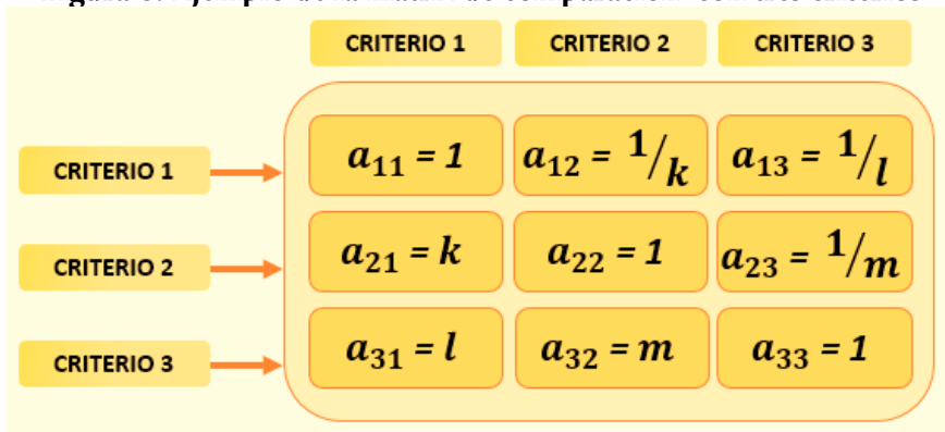
Figura 6. Ejemplo de la matriz de comparación con tres criterios
