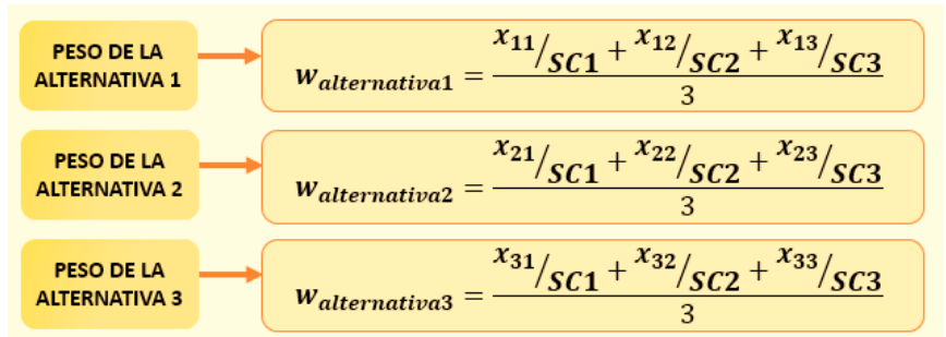
Figura 12. Determinación de los pesos relativos de las alternativas en base a uno de los criterios.
