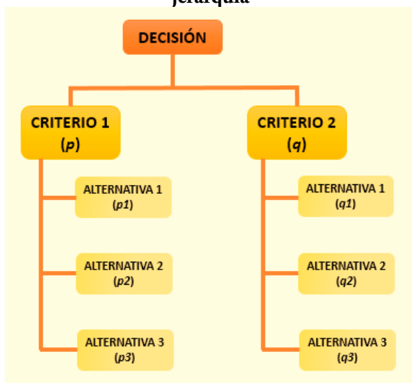
Figura 1. Árbol del Proceso de Jerarquía Analítica con un nivel de jerarquía
