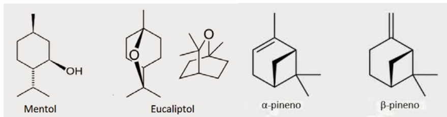
Fig. 6. Ingredientes antivirales de Mentisan®: mentol, eucaliptol, alfa-pineno y beta-pineno, autorización de reproducción pendiente, no se encontraron advertencias de copyright en internet / Mentisan® antiviral ingredients: menthol, eucalyptol, alpha-pinene and beta-pinene, reproduction authorization pending, no copyright notices found on line
