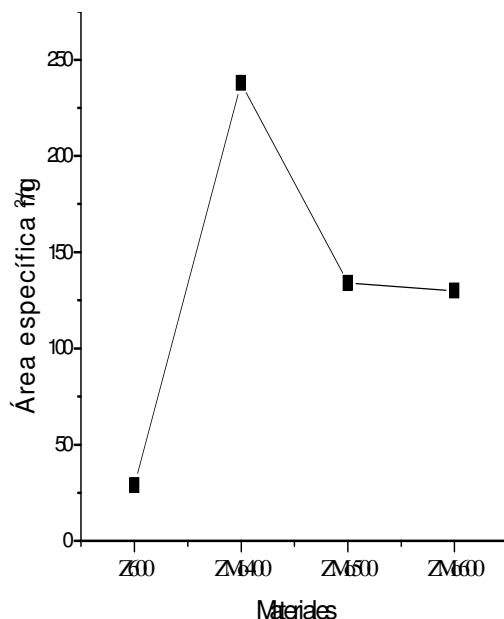
Figura 1. Efecto de la temperatura de calcinación sobre el área específica de la circonia modificada con molibdeno
