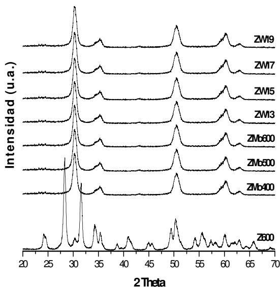
Figura 3. Difractogramas de las muestras ZrO_2 , ZrO_2-MoO_3 y ZrO_2-WO_3
