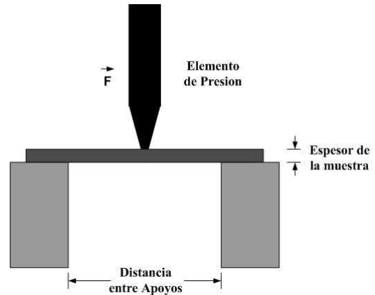
FIG. 3.— Esquema del equipo utilizado durante los ensayos.
