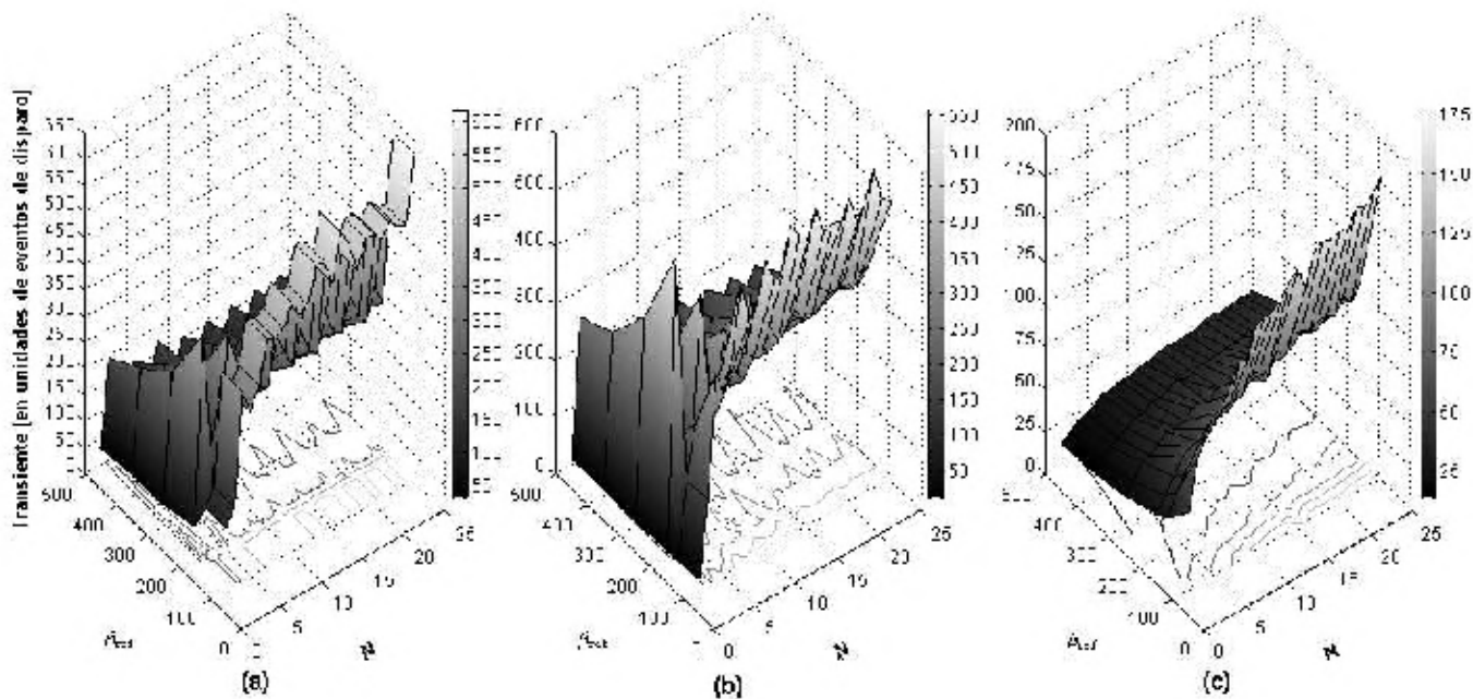
Figura 3. Transiente en función de \beta_{ref} y N para (a) LCOs, (b) LCOs simplificados, y (c) IFOs utilizando el CDF.
