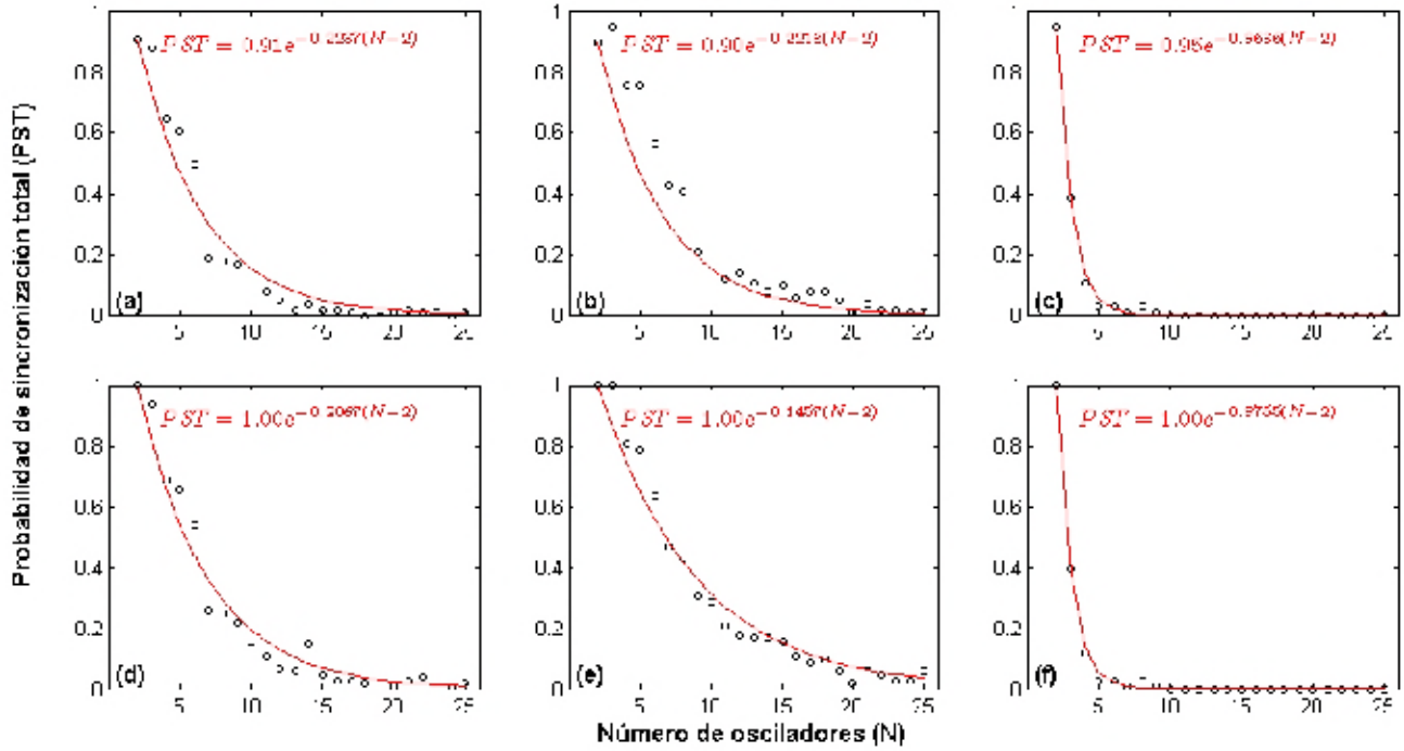
Figura 6. Resultados de la PST utilizando el CDF (arriba) y el CP (abajo) para LCOs (a) y (d), LCOs simplificados (b) y (e) e IFOs (c) y (f). La ecuación de ajuste se muestra para cada caso y la gráfica de la función correspondiente está representada por la línea continua.
