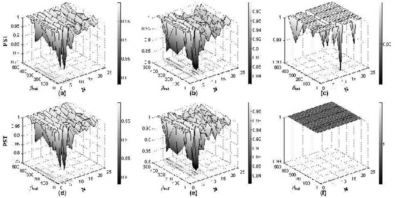
Figura 2. PST en función de \beta_{ref} y N para LCOs (a) y (d), para LCOs simplificados (b) y (e), y para IFOs (c) y (f); utilizando el CDF (a)–(c) y el CP (d)–(f).
