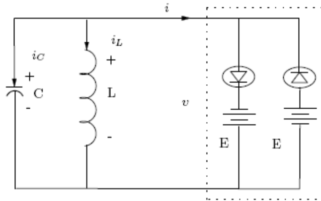
Figura 1: Circuito oscilatorio básico
