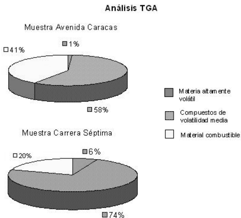
Figura 4: Contenido de material altamente volátil, volatilidad media y material combustible de las muestras de MP recolectadas en la avenida Caracas y en la carrera Séptima.
