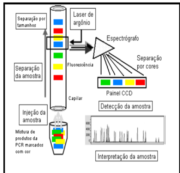
Fig 1 Esquema das etapas de funcionamento da Eletroforese Capilar em Sequenciador Automático
