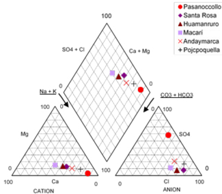
Figura 1. Diagrama de Piper para las muestras de aguas minero medicinales de la provincia de Melgar.
