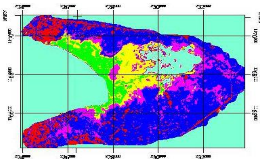
Figura 2. Unidades de paisaje de la Reserva de Fauna Silvestre Ciénaga de La Palmita e Isla de Pájaros. Imagen 058 (2014). LANDSAT 8.
